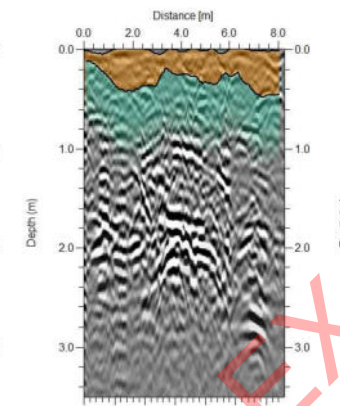
GPR LINE 060
